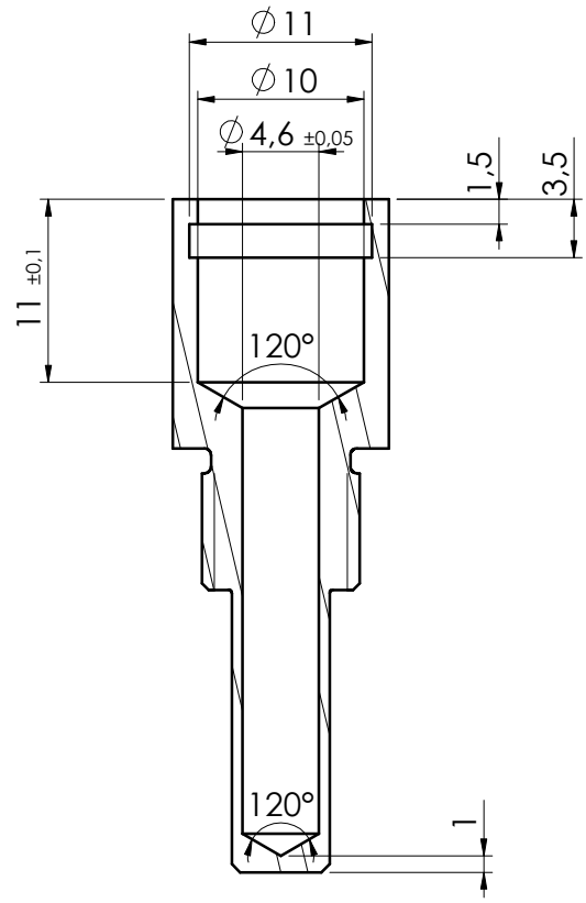
SEZIONE A-A
